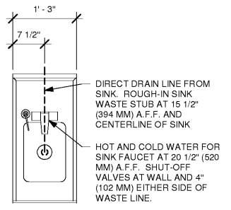
5 ADD 02-01 PLUMBING Scale: 3/4" = 1'-0"
