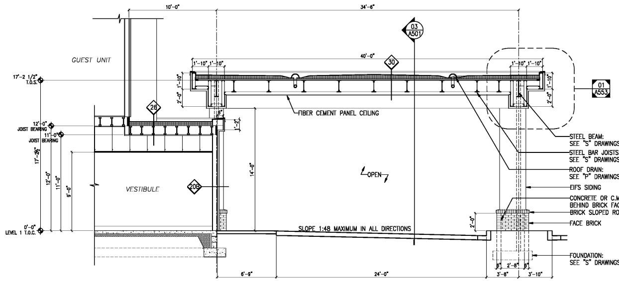
02 PORTE COCHERE
