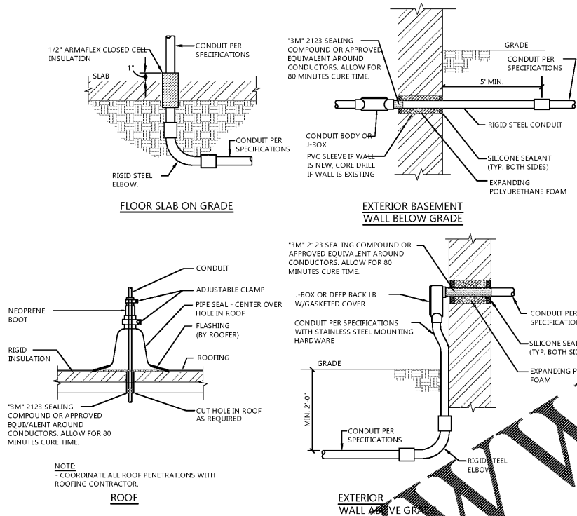
2 CONDUIT PENETRATION DETAIL E3.0 NO SCALE
