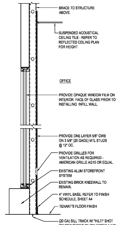
5 SECTION SCALE: 1" = 1'-0"
