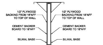
2 CHEF LINE WALL SECTION FS-8.0
