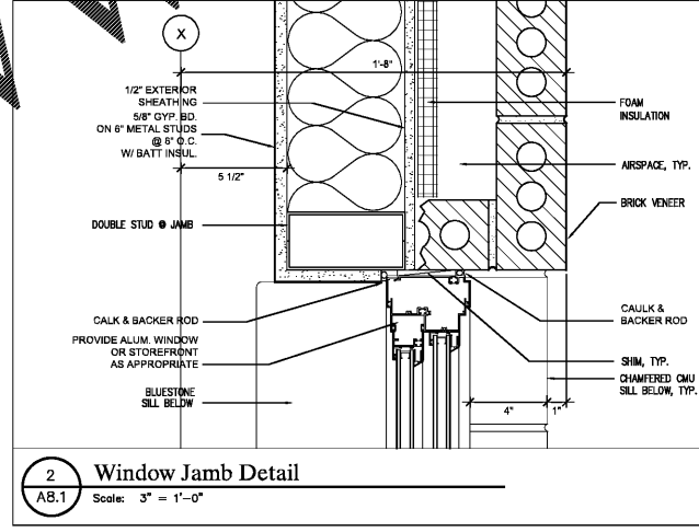
J-2 Jamb Detail AB.1 Scale: 3\"/>
