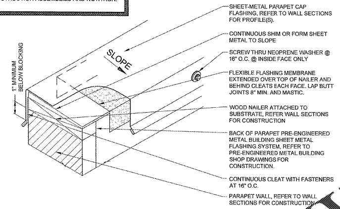
2 TYPICAL COPING FLASHING DETAIL A6.1 SCALE: N.T.S.
