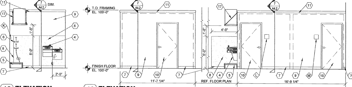
14 ELEVATION A4.1 SCALE: 1/4" = 1'-0" 15 ELEVATION A4.1 SCALE: 1/4" = 1'-0"
