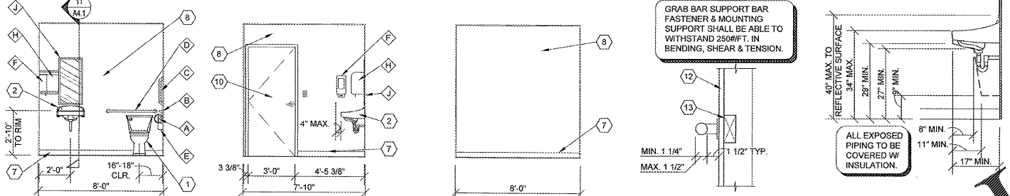
7 ELEVATION A4.1 SCALE: 1/4" = 1'-0" 8 ELEVATION A4.1 SCALE: 1/4" = 1'-0" 9 ELEVATION A4.1 SCALE: 1/4" = 1'-0" 10 ELEVATION A4.1 SCALE: 1/2" = 1'-0" 11 LAVATORY CLEARANCES A4.1 SCALE: 1/2" = 1'-0"
