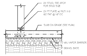
2 SECTION SD-2 SCALE: 1" = 1'-0"
