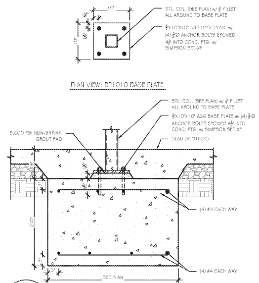
3 SECTION SD-2 SCALE: 1" = 1'-0"
