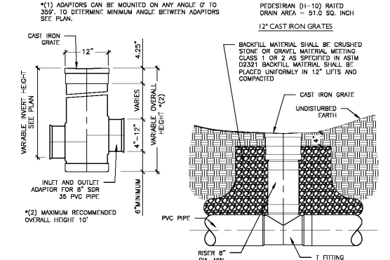
1 Area Inlet Detail N.T.S.
