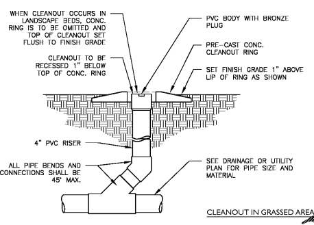
3 Cleanout N.T.S.
