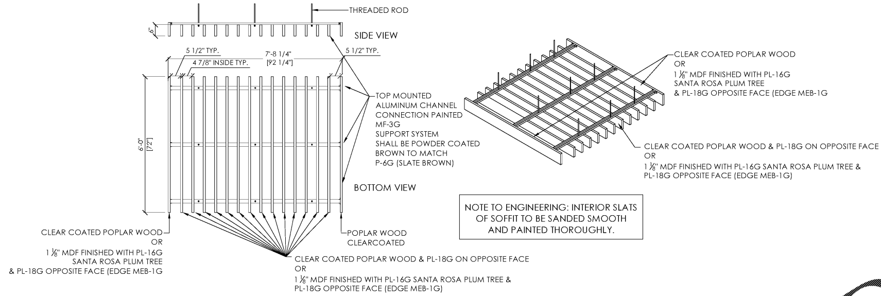
5 PERGOLA DETAIL SCALE: 1/2" = 1'-0"
