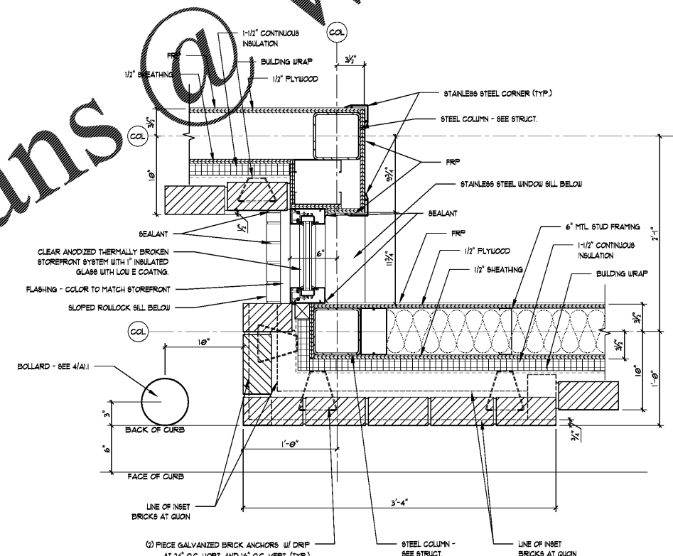
3 PLAN DETAIL (QUON) SCALE: 1 1/2"=1'-0"
