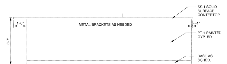
12 ELEVATION A-901 SCALE: 1/2" = 1'-0"
