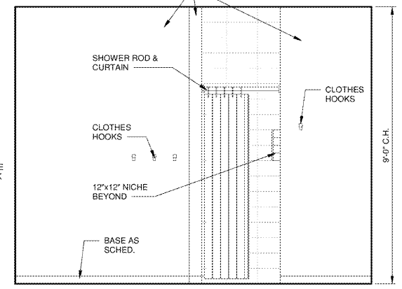
2 ELEVATION A-901 SCALE: 1/2" = 1'-0"
