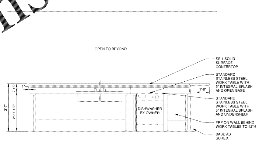
10 ELEVATION A-901 SCALE: 1/2" = 1'-0"
