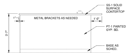
11 ELEVATION A-901 SCALE: 1/2" = 1'-0"
