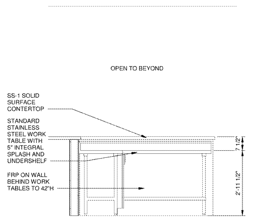
8 ELEVATION A-901 SCALE: 1/2" = 1'-0"
