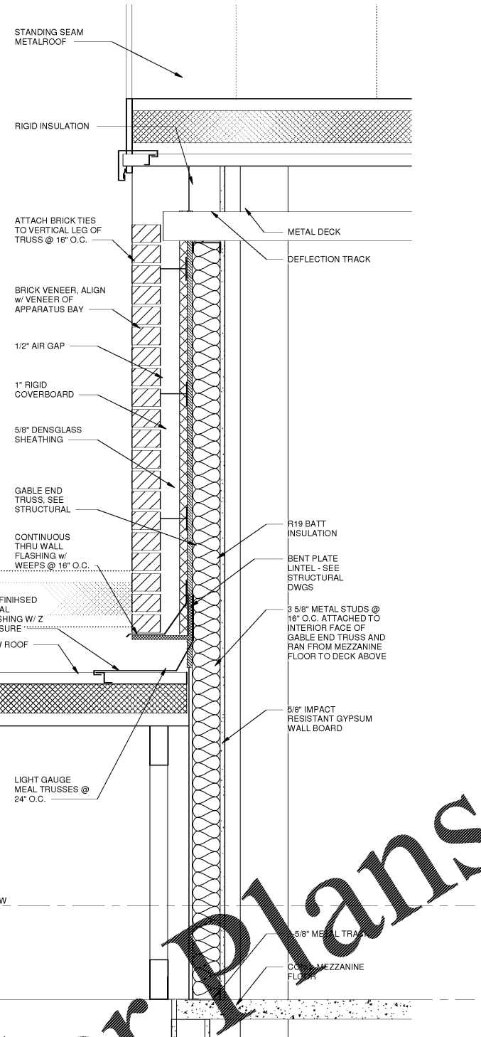
1 SECTION A-602 SCALE: 1/4" = 1'-0"
