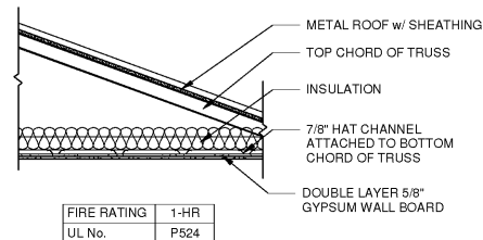
2 A-201 1-HR CEILING ASSEMBLY SCALE: 1/2" = 1'-0"
