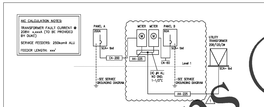
ELECTRICAL RISER PLAN SCALE: NONE
