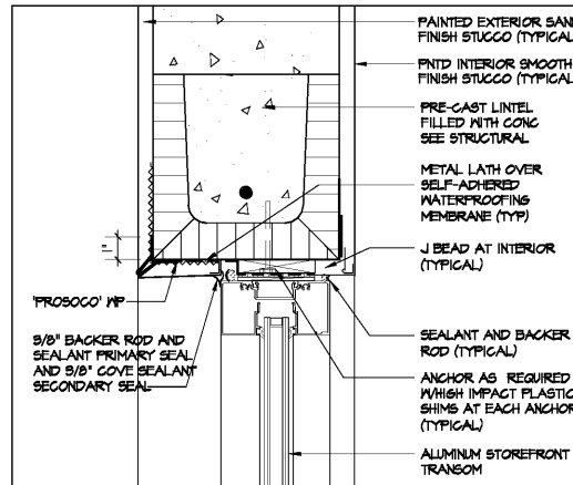
6 STOREFRONT HEAD SCALE: 3" = 1'-0"
