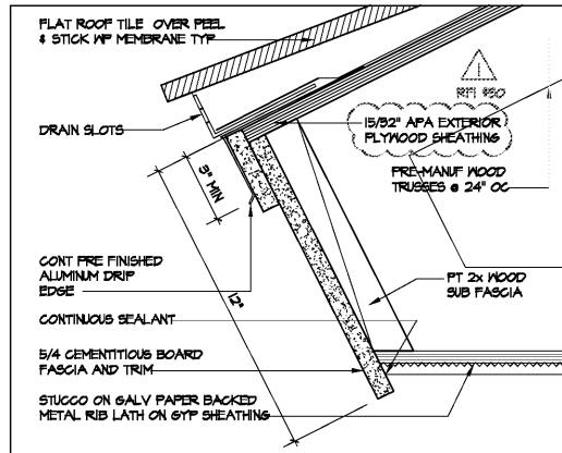
1 FASCIA DETAIL SCALE: 3" = 1'-0"
