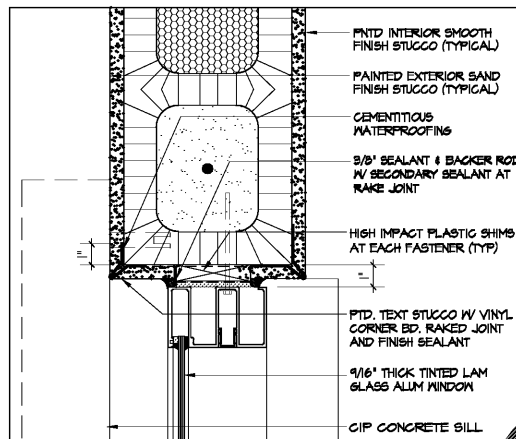
9 FIXED WINDOW JAMB SCALE: 3" = 1'-0"
