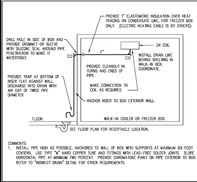
5 CONDENSATE DRAIN (WALK-IN BOX)
