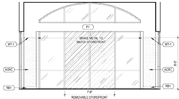
3 FRONT VESTIBULE ELEV. A10.1 1/4" = 1'-0"
