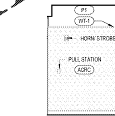
7 REAR VESTIBULE ELEV. A10.1 1/4" = 1'-0"
