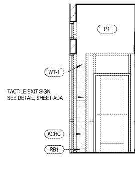
4 FRONT VESTIBULE ELEV. A10.1 1/4" = 1'-0"
