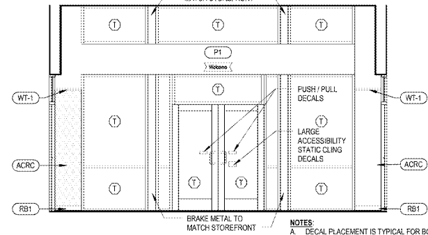
2 FRONT VESTIBULE ELEV. A10.1 1/4" = 1'-0"
