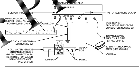
2 GROUNDING ELECTRODE SYSTEM DETAIL SCALE: N.T.S.
