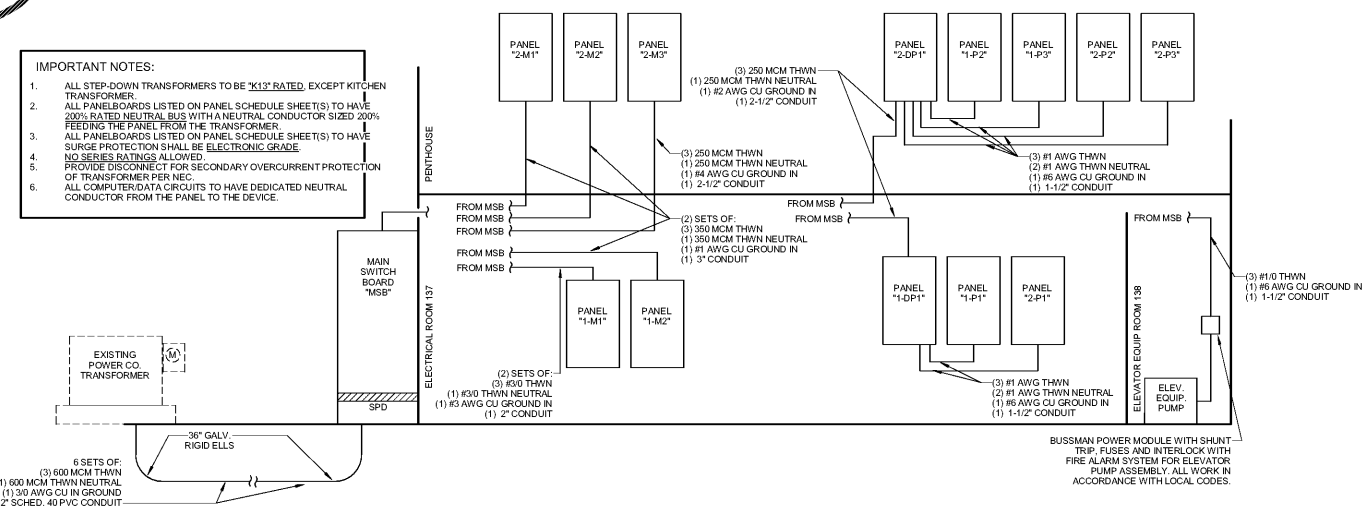
1 ELECTRICAL RISER DIAGRAM - SYSTEM 1 SCALE: N.T.S.
