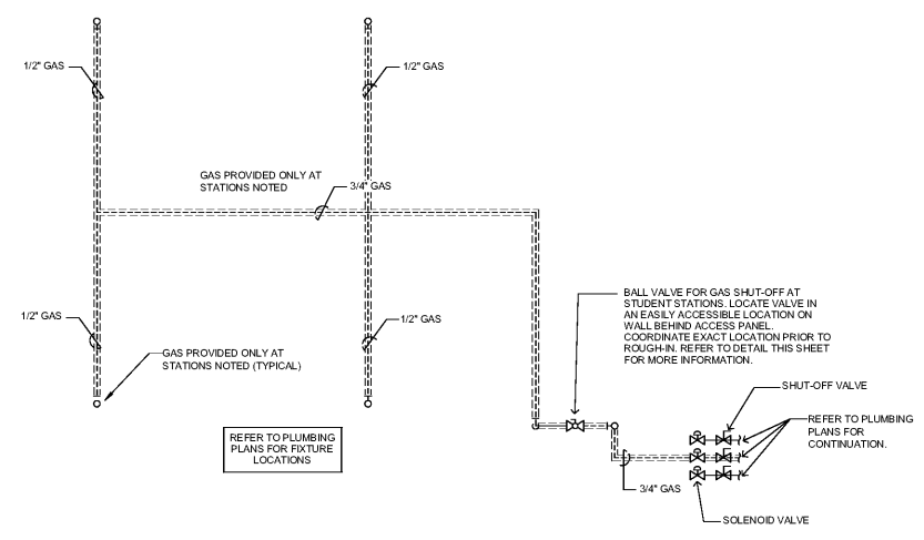
1 SCIENCE LAB GAS SUPPLY - SCHEMATIC DIAGRAM SCALE: N.T.S.
