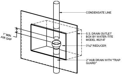
13 CONDENSATE HUB DRAIN DETAIL SCALE: N.T.S.
