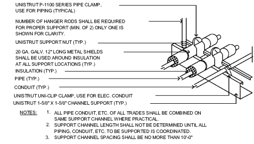
11 PIPING SUPPORT ABOVE CEILING DETAIL SCALE: N.T.S.
