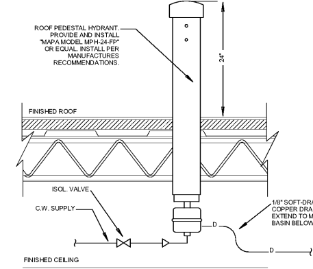
10 NON FREEZE ROOF HYDRANT SCALE: N.T.S.
