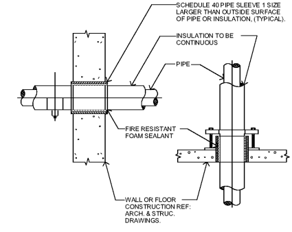
9 PIPE SLEEVE DETAILS SCALE: N.T.S.
