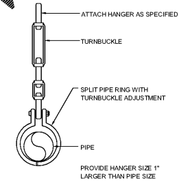
6 PIPE HANGER DETAIL SCALE: N.T.S.
