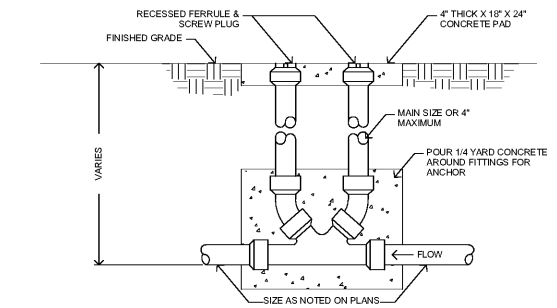
2 TWO-WAY GRADE CLEANOUT DETAIL SCALE: N.T.S.
