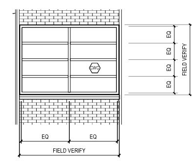
3 CURTAINWALL - CWC A3.4 SCALE: 3/8" = 1'-0"
