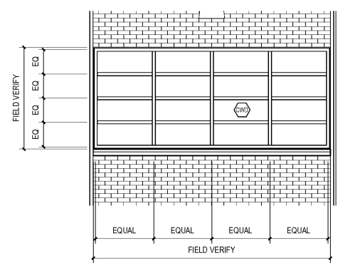
4 CURTAINWALL - CWD A3.4 SCALE: 3/8" = 1'-0"
