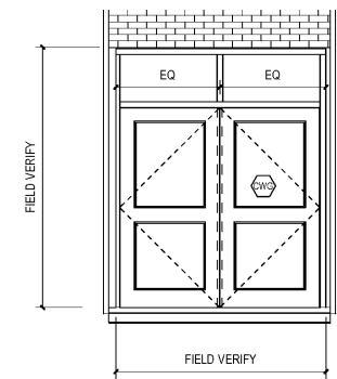
7 CURTAINWALL - CWG A3.4 SCALE: 3/8" = 1'-0"
