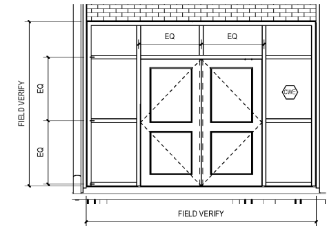
5 CURTAINWALL - CWE A3.4 SCALE: 3/8" = 1'-0"
