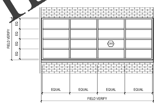
2 CURTAINWALL - CWB A3.4 SCALE: 3/8" = 1'-0"
