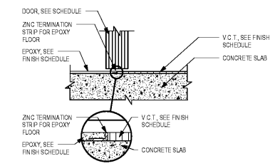
2 SILL -- EPOXY - V.C.T. A3.3 SCALE: 3" = 1'-0"
