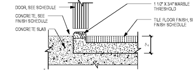
7 SILL -- CONCRETE - TILE A3.3 SCALE: 3" = 1'-0"
