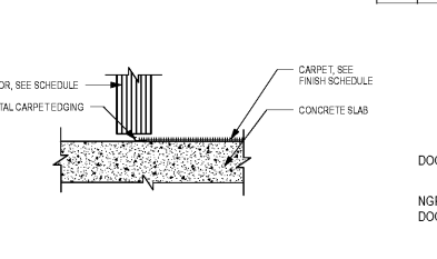
5 SILL -- CONCRETE - CARPET A3.3 SCALE: 3" = 1'-0"
