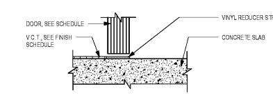
6 SILL -- CONCRETE - V.C.T. A3.3 SCALE: 3" = 1'-0"
