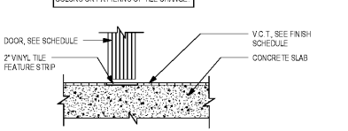
9 SILL -- V.C.T. - V.C.T. A3.3 SCALE: 3" = 1'-0"
