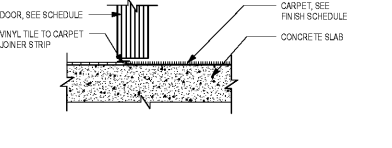
8 SILL -- V.C.T. - CARPET A3.3 SCALE: 3" = 1'-0"
