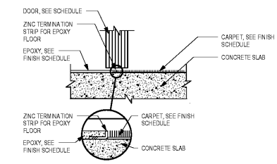
1 SILL -- EPOXY - CARPET A3.3 SCALE: 3" = 1'-0"
