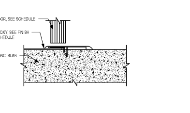
4 SILL -- CONCRETE - EPOXY A3.3 SCALE: 3" = 1'-0"
