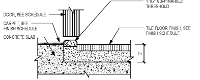
12 SILL -- TILE - CARPET A3.3 SCALE: 3" = 1'-0"
