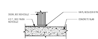
11 SILL -- V.C.T. - CONCRETE A3.3 SCALE: 3" = 1'-0"
