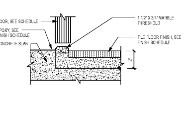
3 SILL -- EPOXY - TILE A3.3 SCALE: 3" = 1'-0"
