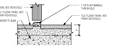
13 SILL -- TILE - TILE A3.3 SCALE: 3" = 1'-0"
