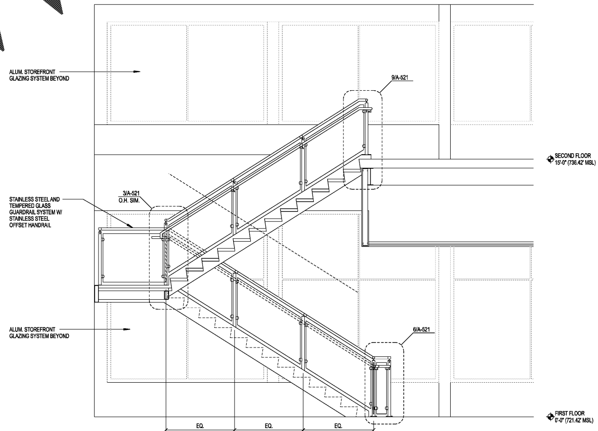
3 A-421 STAIR SECTION
