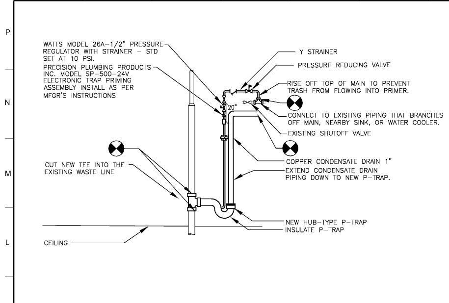
DETAIL - CONDENSATE DRAIN TRAP - NEW SCALE: NONE 1
