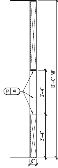
R1.1 SECTION ID.613 SCALE: 1/2" = 1'-0"
