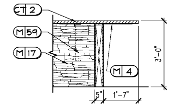
C3.1 SECTION ID.603 SCALE: 1/2" = 1'-0"
