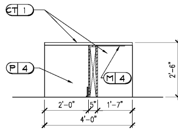
A3.1 SECTION D.600 SCALE: 1/2" = 1'-0"
