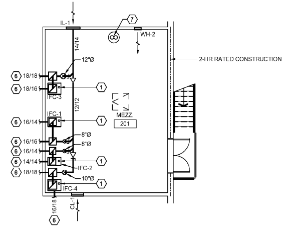
② MEZZANINE HVAC PLAN M-101 SCALE: 1/8" = 1'-0"
