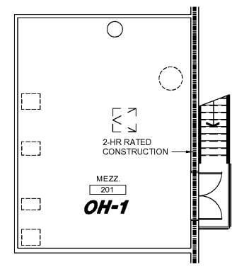
② MEZZANINE FIRE PROTECTION PLAN SCALE: 1/8" = 1'-0"
