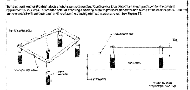
S. R. SMITH multiLIFT™ ANCHOR BONDING DETAIL N.T.S.
