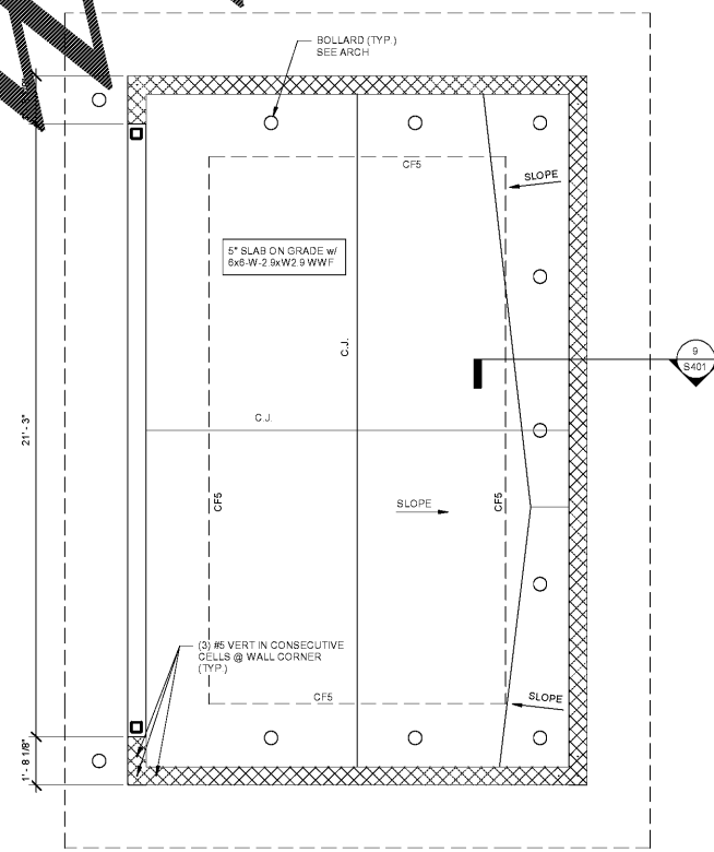
8 DUMPSTER ENCLOSURE S401 SCALE: 3/8" = 1'-0"
