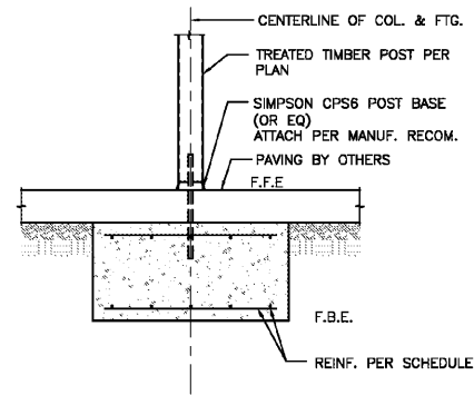
A SECTION S2.2 SCALE: 1/2" = 1'-0"
