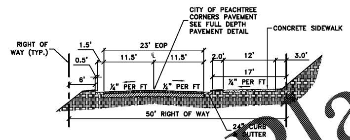
TYPICAL CROSS SECTION A-A: STA 100+40 TO STA 101+00 SCALE: 1"=10'
