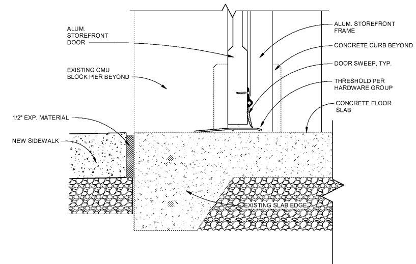
S4 S.F. DOOR SILL SCALE: 3" = 1'-0"
