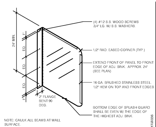
SPLASH GUARD N.T.S. 11
