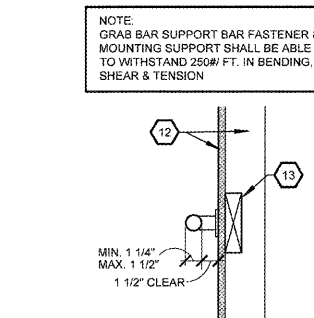
15 GRAB BAR DETAIL A4.1 SCALE: 1 1/2" = 1'-0"
