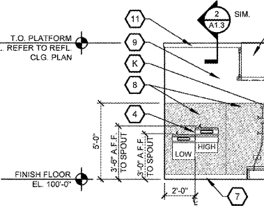
11 ELEVATION A4.1 SCALE: 1/4" = 1'-0"
