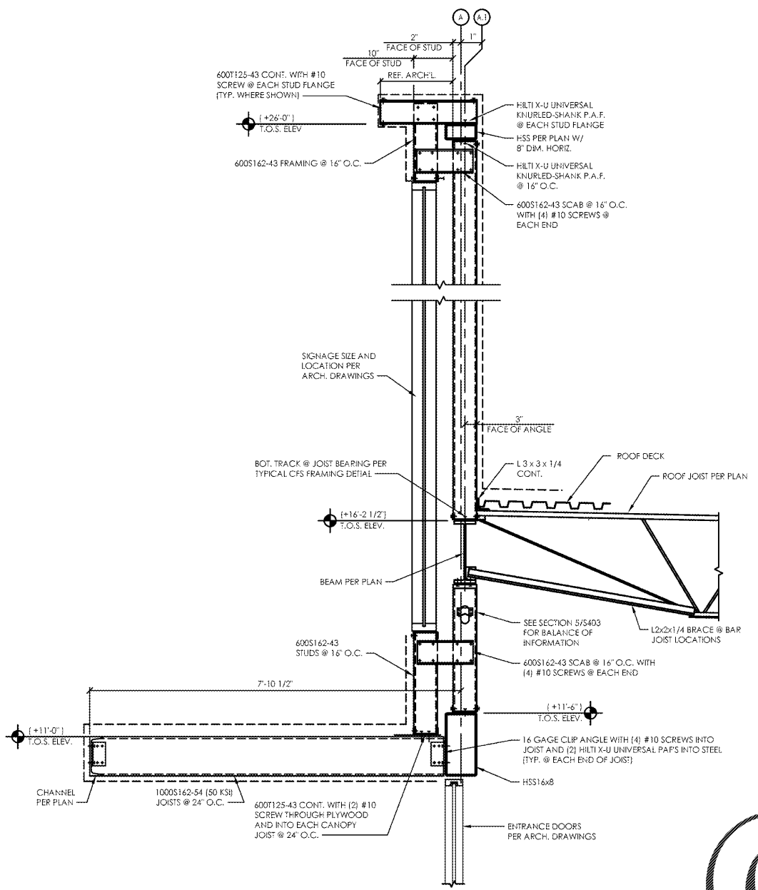
1 Section SCALE: 3/4" = 1'-0"
