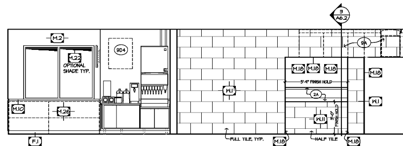
2 ELEVATION
