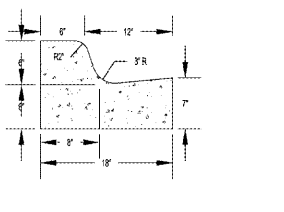
WAWA TYPE F1 CURB NTS
