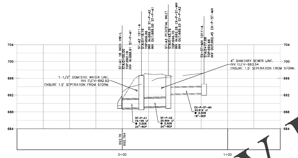
STORM A VERTICAL SCALE: 5.00 HORIZONTAL SCALE: 20.00
