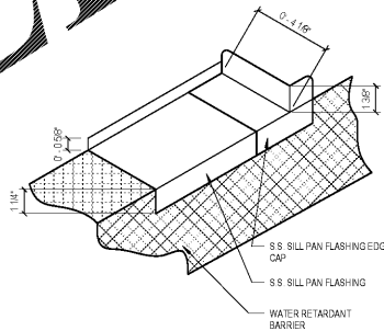
9 Sill Pan Flashing Detail SCALE: 3" = 1'-0"
