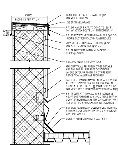
2 Parapet Detail SCALE: 3/4" = 1'-0"
