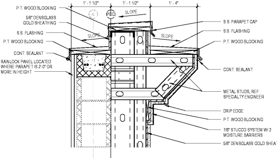
3 Cornice Profile 'C' SCALE: 1" = 1'-0"
