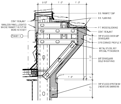
1 Cornice Profile 'A' SCALE: 1" = 1'-0"
