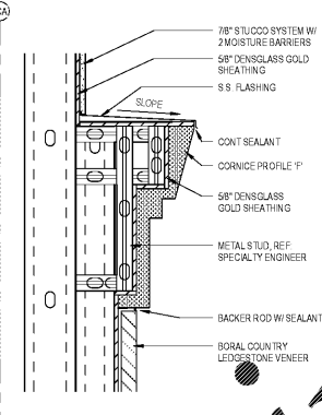
5 Cornice Profile 'F' SCALE: 1" = 1'-0"
