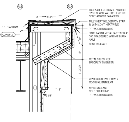
2 Cornice Profile 'B' SCALE: 1" = 1'-0"
