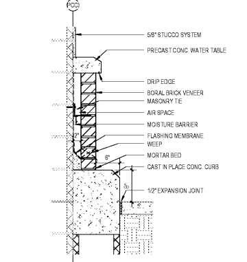
19 Base Detail SCALE: 1" = 1'-0"
