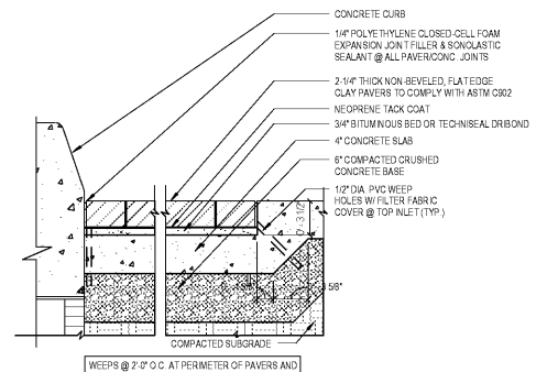
13 Paver Detail SCALE: 1 1/2" = 1'-0"
