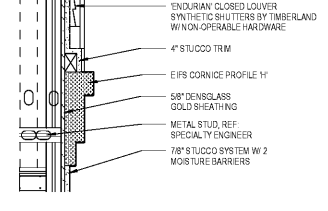
8 Trim Detail SCALE: 1" = 1'-0"
