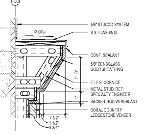
4 Cornice Profile 'D' SCALE: 1" = 1'-0"
