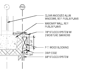
16 Trim Detail SCALE: 1 1/2" = 1'-0"
