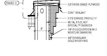
9 Parapet Detail SCALE: 1" = 1'-0"
