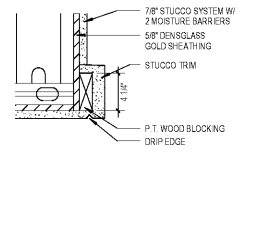
12 Trim Detail SCALE: 1 1/2" = 1'-0"
