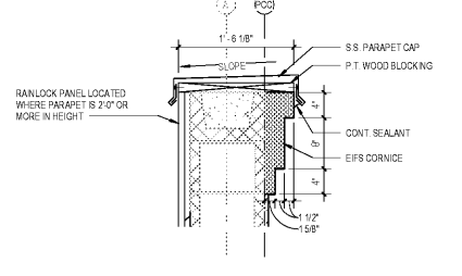
7 Cornice Profile 'H' SCALE: 1" = 1'-0"
