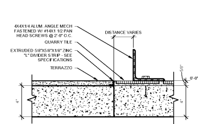
2 CASE ANGLE SCALE: 3" = 1'-0"
