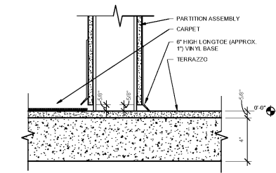
1 CARPET OVER TERRAZZO SCALE: 3" = 1'-0"
