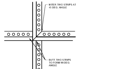
11 TERRAZZO METAL STRIPS SCALE: 6" = 1'-0"
