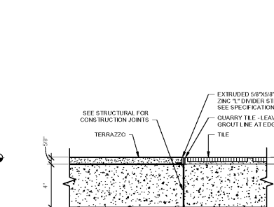
19 TERRAZZO TO TILE SCALE: 3" = 1'-0"
