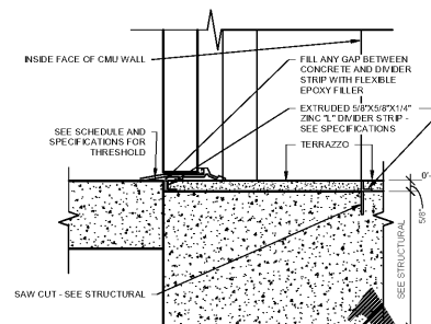
16 TERRAZZO TO EXTERIOR DOOR SCALE: 3" = 1'-0"
