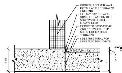
15 TERRAZZO TO COOLER WALL SCALE: 3" = 1'-0"
