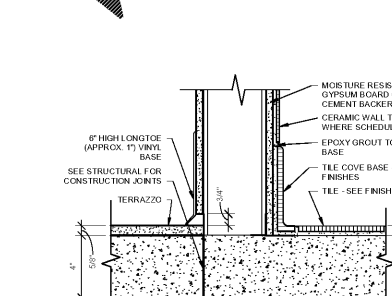
18 TERRAZZO TO STUD WALL SCALE: 3" = 1'-0"
