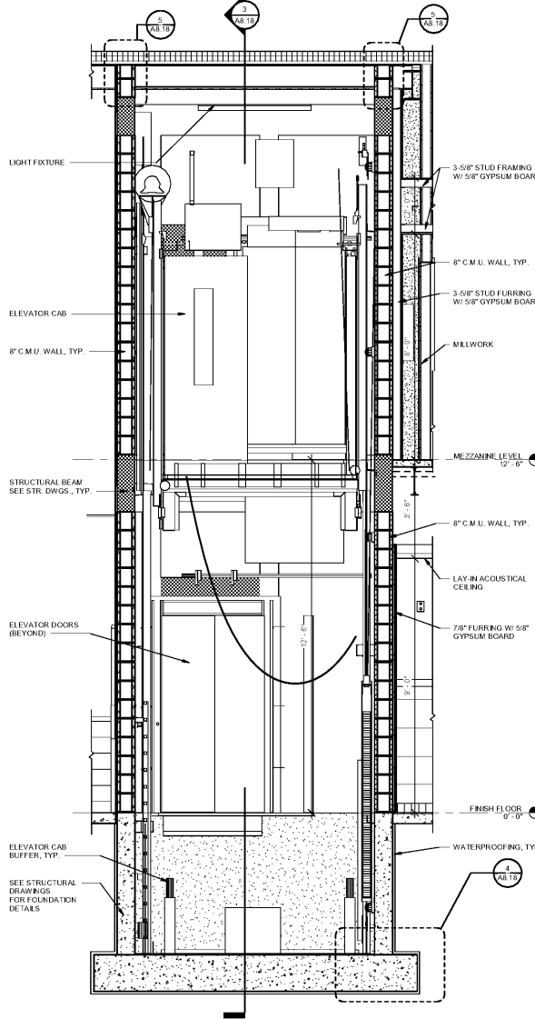
ELEVATOR SECTION SCALE: 1/2" = 1'-0"
