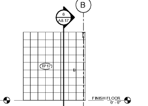
10 OMNI CHANNEL SCALE: 1/4" = 1'-0"
