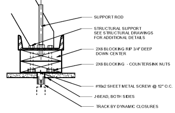
9 PHARMACY ROLLING GRILLE HEADER SCALE: 3" = 1'-0"
