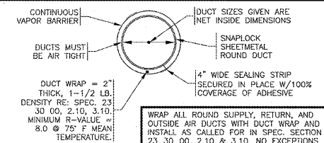
ROUND DUCT WRAP INSULATION N.T.S.
