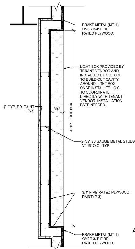
4 ENLARGED STOREFRONT DETAIL A202 SCALE: 1-1/2" = 1'-0"
