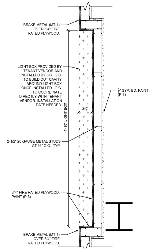
3 ENLARGED STOREFRONT DETAIL A202 SCALE: 1-1/2" = 1'-0"
