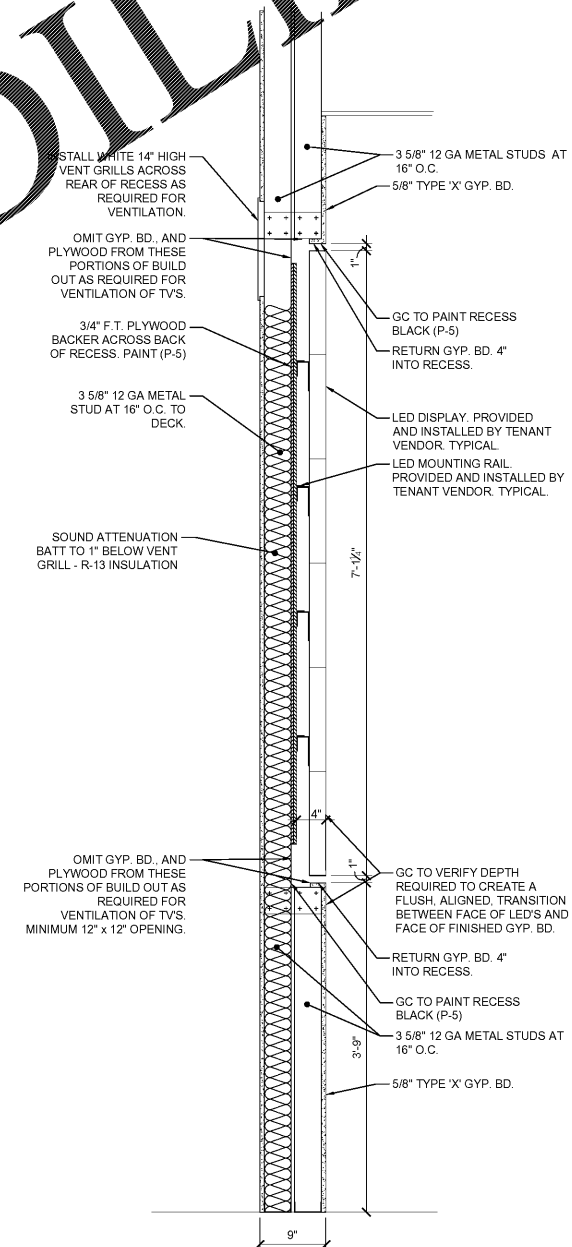
2 WALL TYPE 'B3' A202 SCALE: 1" = 1'-0"
